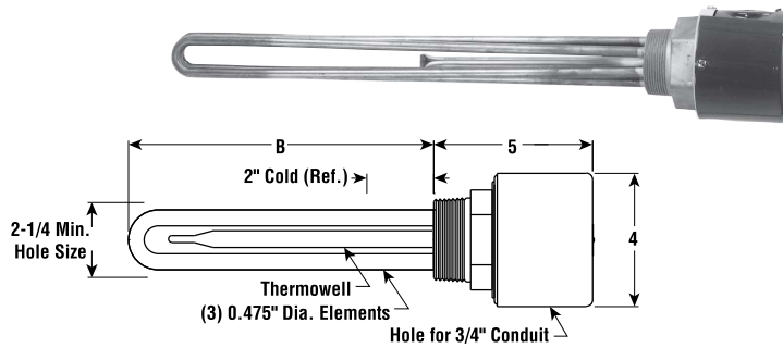
E2 — Dimensions (Inches)
