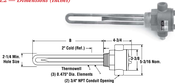
E2 — Dimensions (Inches)
