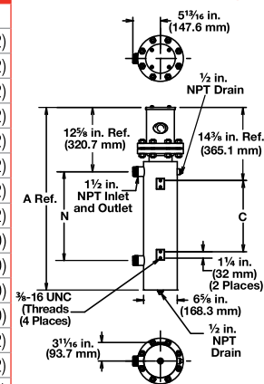
4 inch - 150 lb ANSI Flange
