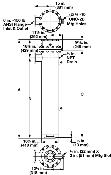
14 inch - 150 lb ANSI Flange
