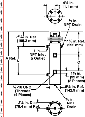
3 inch - 150 lb ANSI Flange
