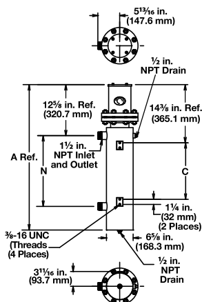
4 inch - 150 lb ANSI Flange
