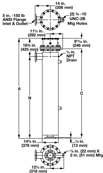
12 inch - 150 lb ANSI Flange
